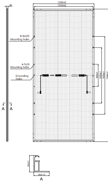
태양광 모듈 치수 Unit: mm
